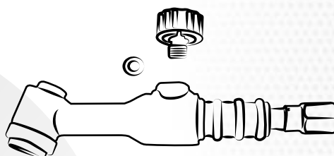
Гусак горелки с клапаном
